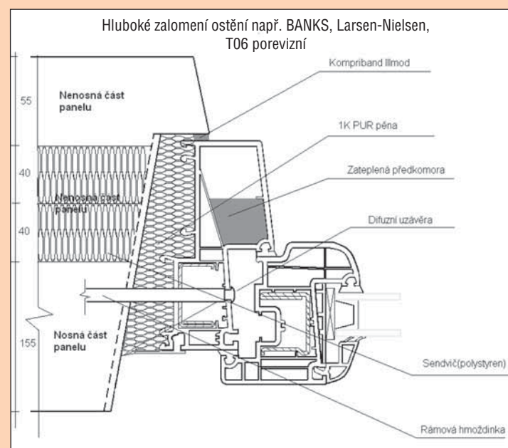
Kotvení rámu okna mimo prostor sendviče, do nosné části panelu. Provedení oken systém SULKO HR+, připojovací spára S3, montáž suchou cestou.
